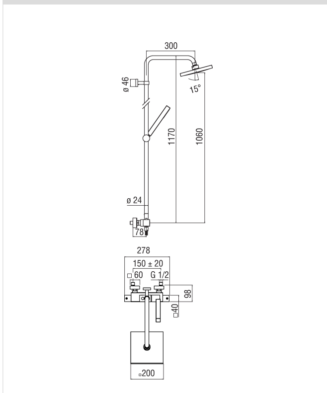
Dessin technique
