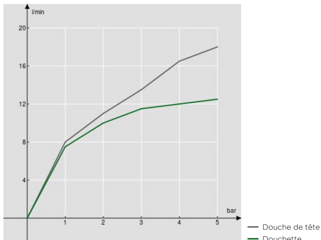
GRAPHIQUE DE DÉBIT: CHAUDE/FROIDE
