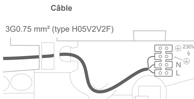
fig. 26 - Remplacement du câble d'alimentation
