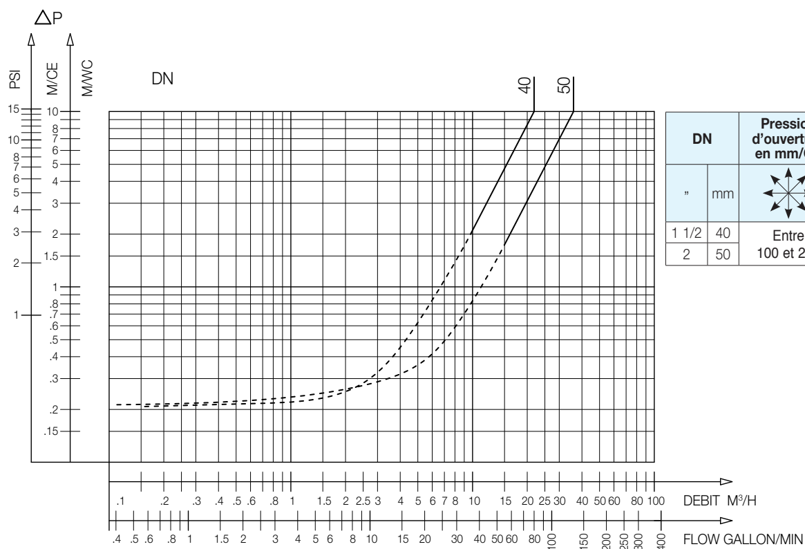
190 - Abaque des pertes de charge
