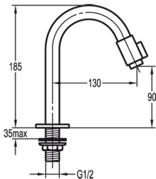
Schéma technique
