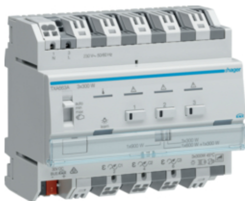
Module 3 sorties variation 300W / NE
